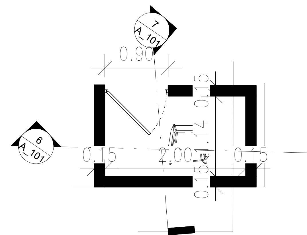
PLANTA GARITA DE SEGURIDAD 2
