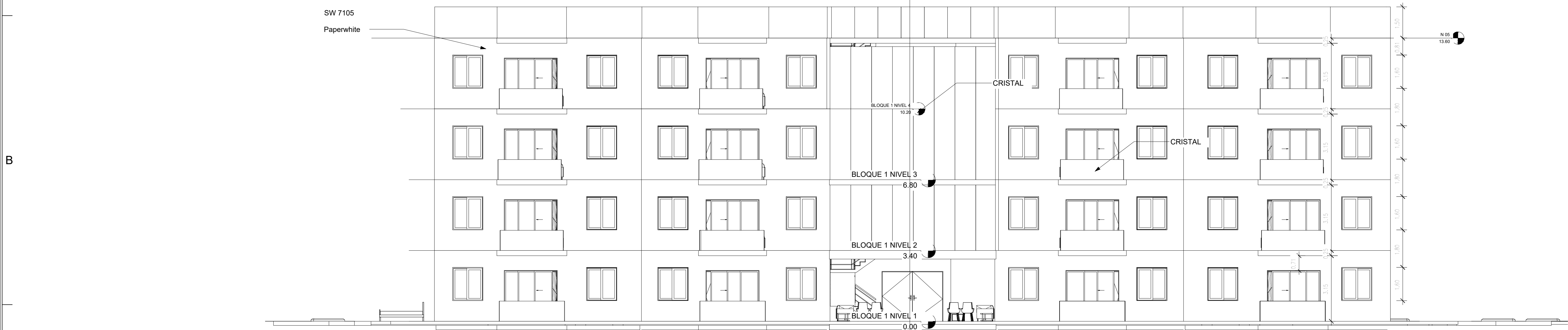
ELEVACION POSTERIOR BLOQUE 1 ESCALA 1:100
