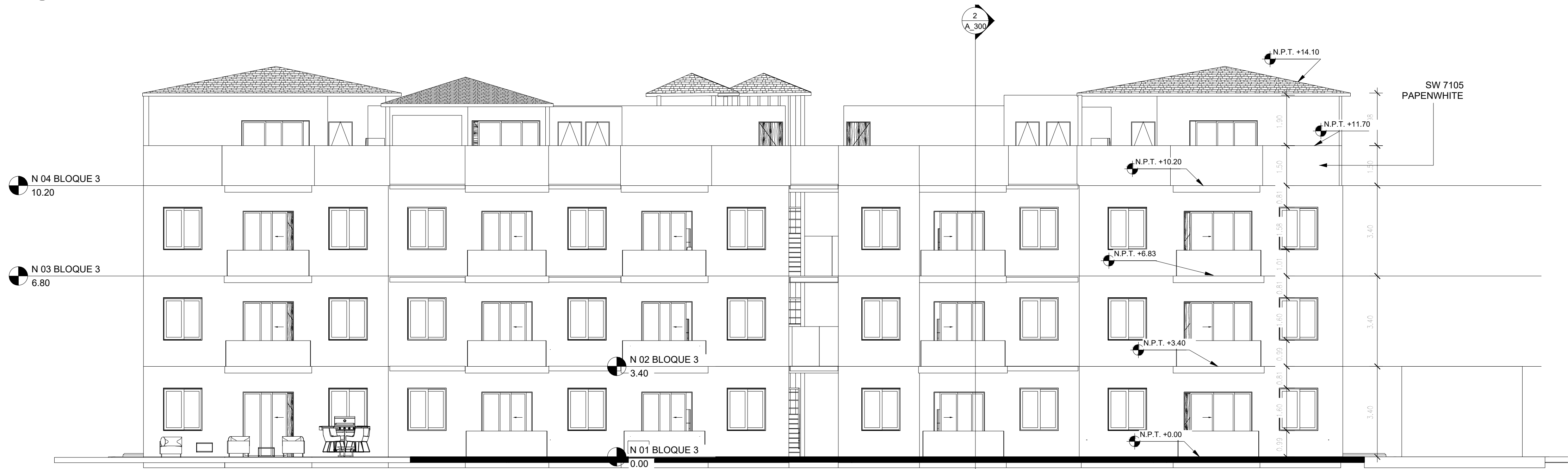
ELEVACION FRONTAL BLOQUE 3 ESCALA 1:100
