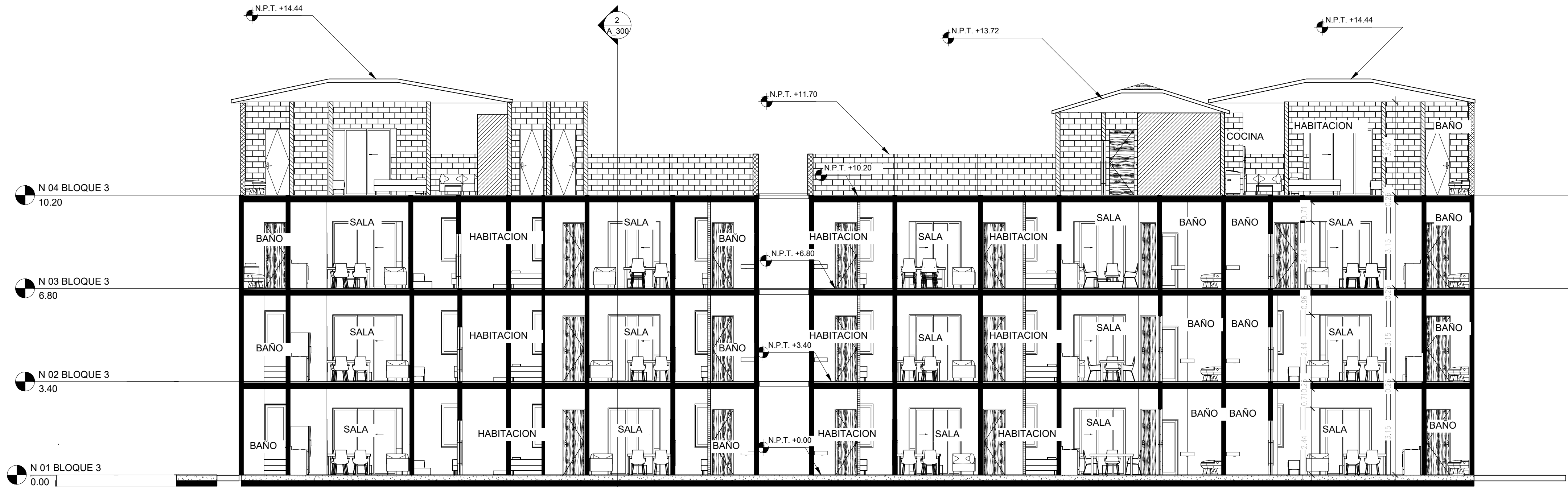
SECCION LONGITUDINAL BLOQUE 4 ESCALA 1:100
