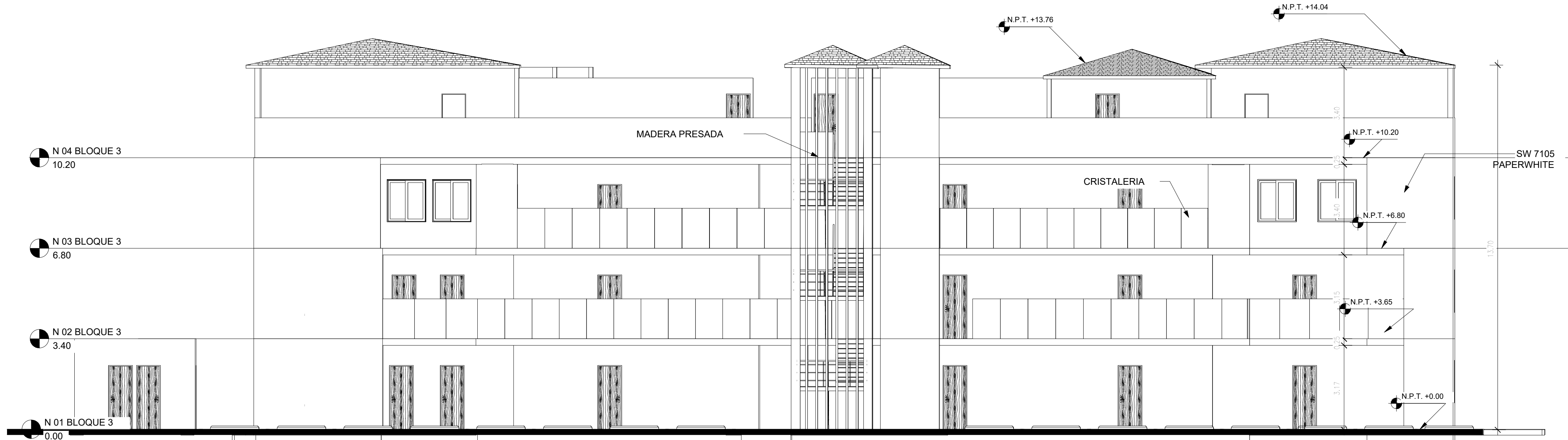
ELEVACION FRONTAL BLOQUE 3 ESCALA 1:100
