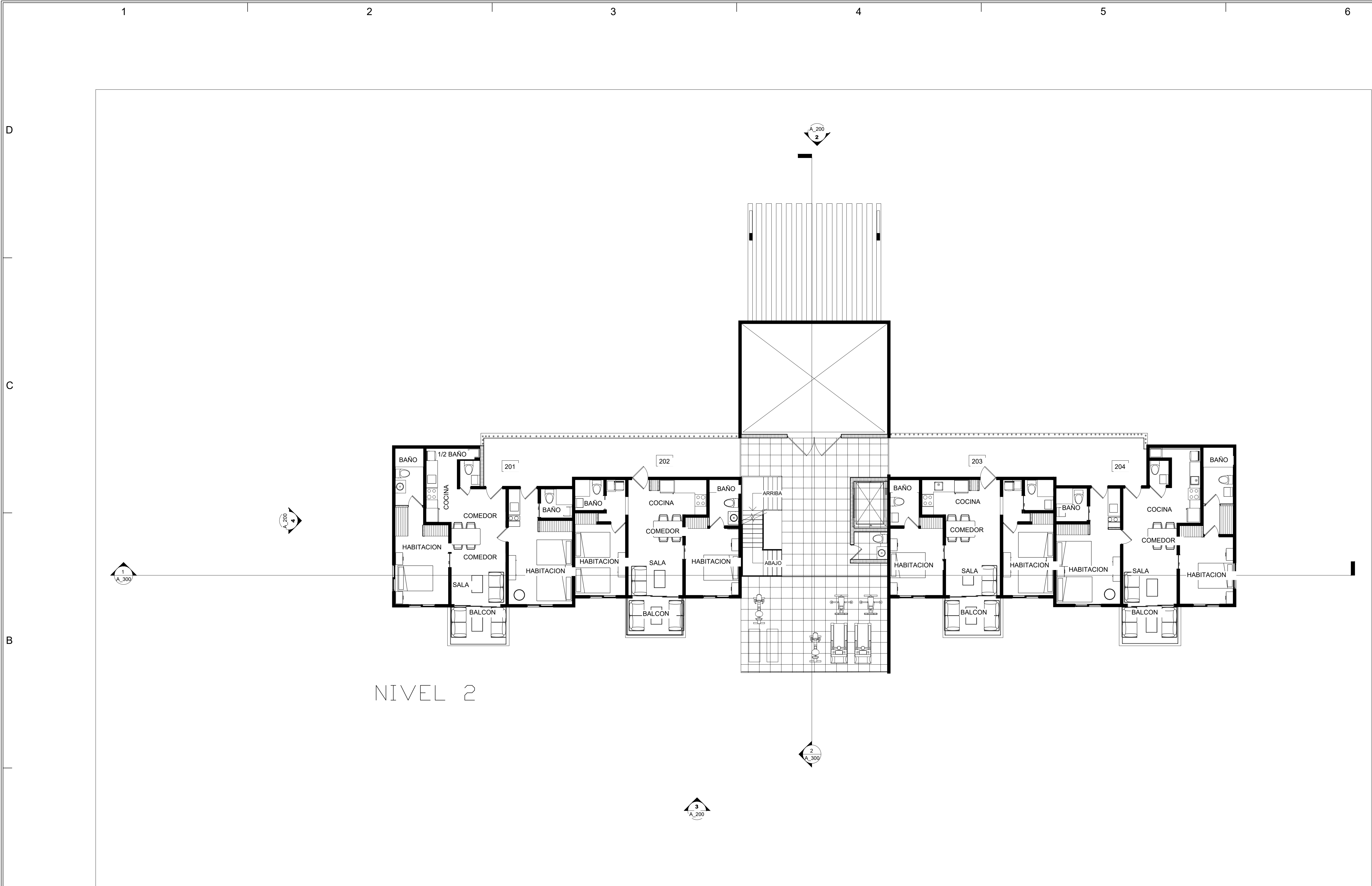
PLANTA ARQUITECTONICA BLOQUE 1 NIVEL 2 ESCALA 1:75
