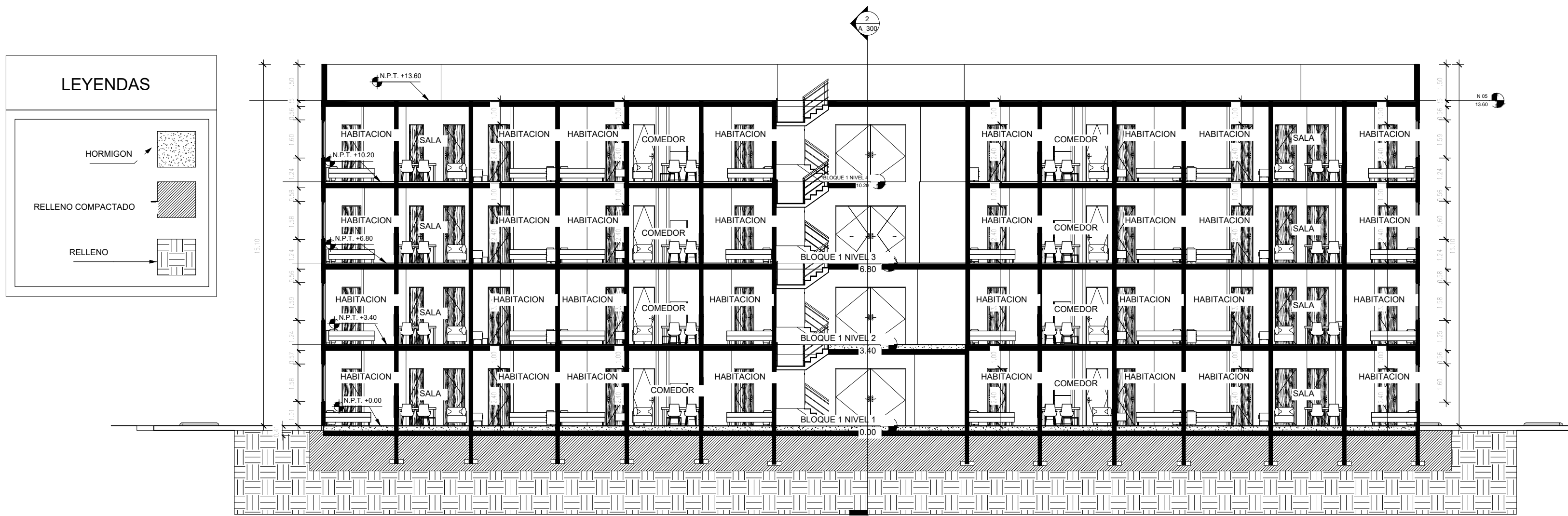
SECCION TRANSVERSAL BLOQUE 1 ESCALA 1:100
